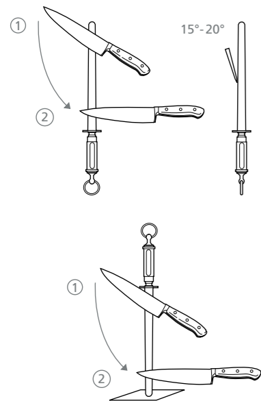
Wetzstahl senkrecht auf eine Unterlage
