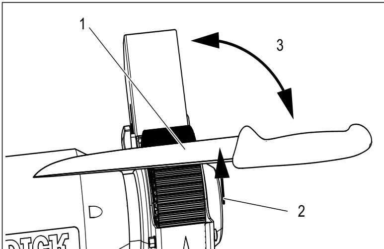
Bild 8.1 – Messer schleifen
